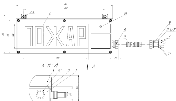
Рисунок 1. Внешний вид оповещателя.
